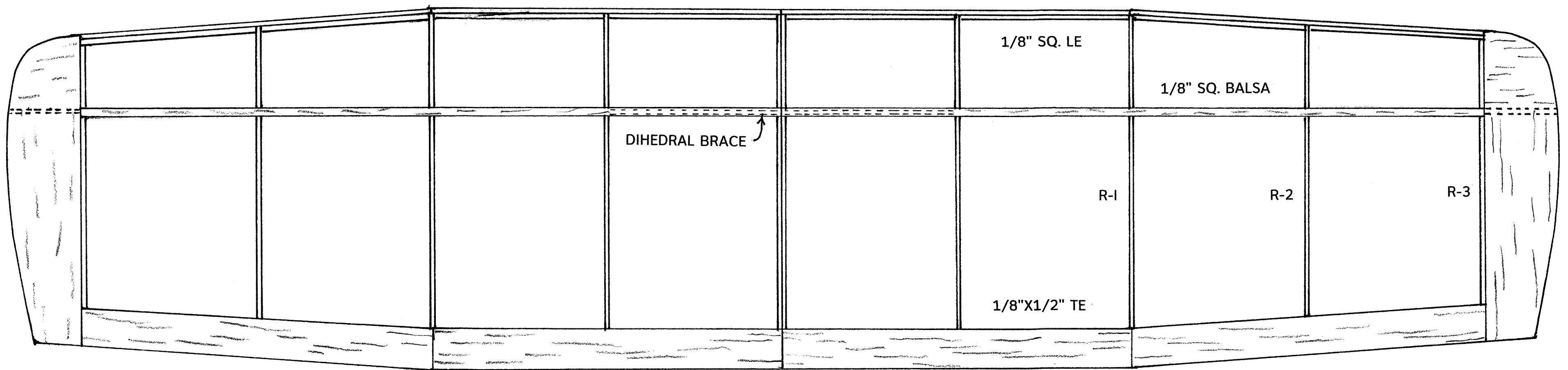
1/16" Balsa Brace
